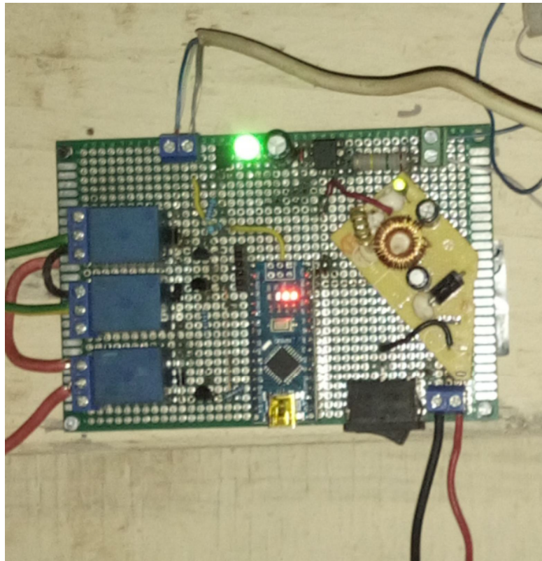
Модель системи віддаленого керування
