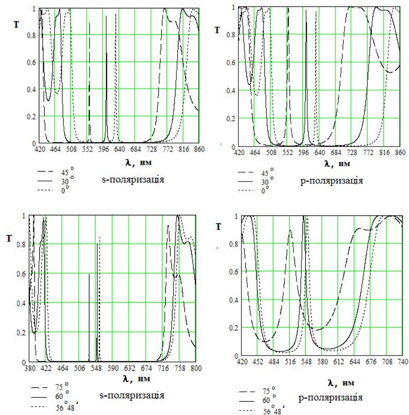
РИС. 2. Трансформація спектрів пропускання вузькосмугового фільтра з робочою довжиною хвилі \lambda_0 = 630 нм зі зміною кутів падіння.
